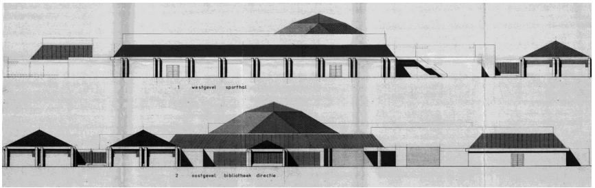
Gevels MOC: west- en oostgevel
